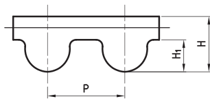
HTD8M TP
