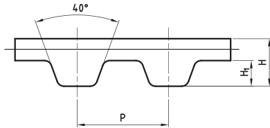
T10 TP
