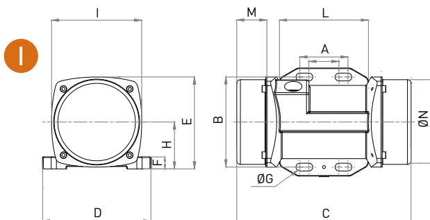
DIMENSIONI DI INGOMBRO (mm)
