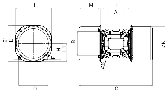
DIMENSIONI DI INGOMBRO (mm)
