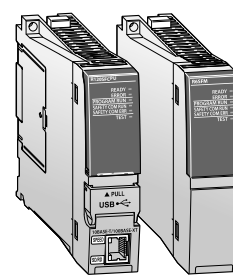
R120SFCPU/R6SFM CPU di sicurezza e modulo funzione di sicurezza
