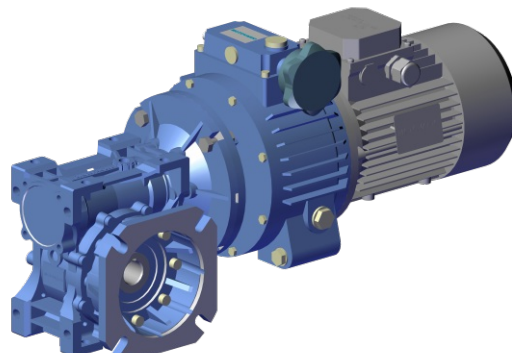
TXF.../SF...+NMRV030F/130F
