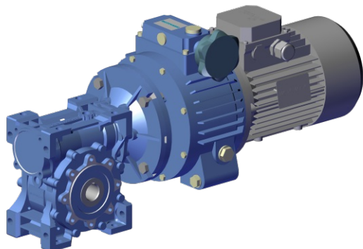
TXF.../SF...+NMRV030/130
