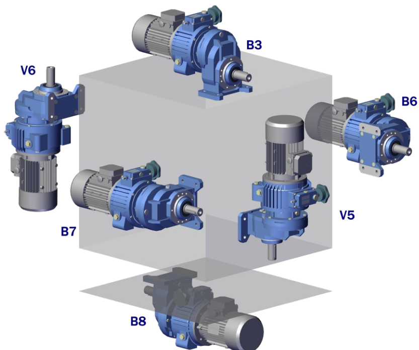
VHM.../A.1 - VHRM.../..1
